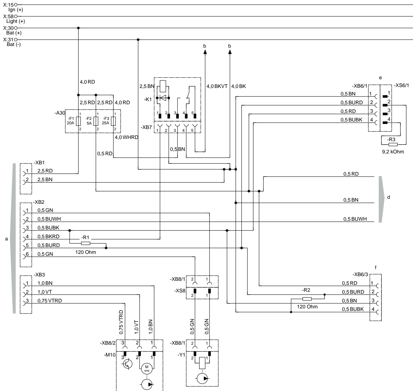
МОНТАЖНАЯ СХЕМА КАБЕЛЬНОГО ЖГУТА
